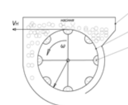
Рис. 1. Назва рисунка: 1 - корпус висівного апарату; 2- котушка; 3- насіння
